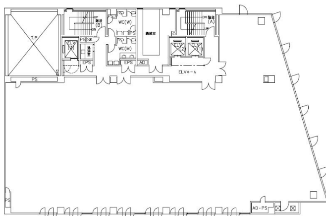
基準階平面図
